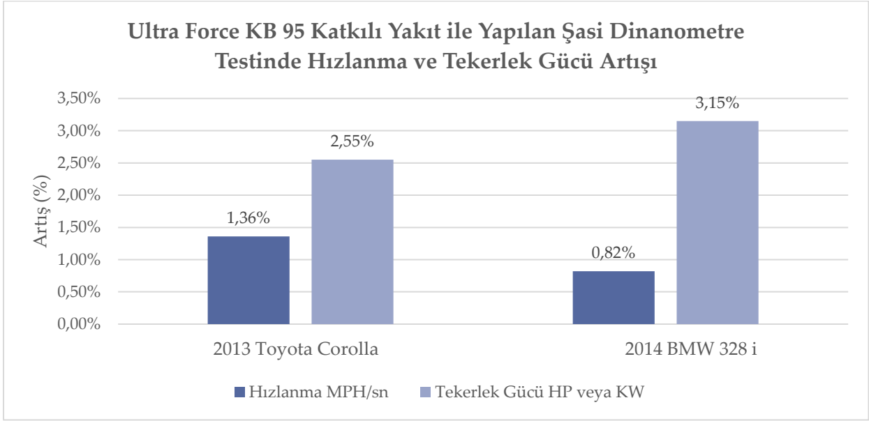
Şekil 4 Ultra Force KB 95 Katkılı Yakıt ile Yapılan Şasi Dinanometre Testinde Hızlanma ve Tekerlek Gücü Artışı
