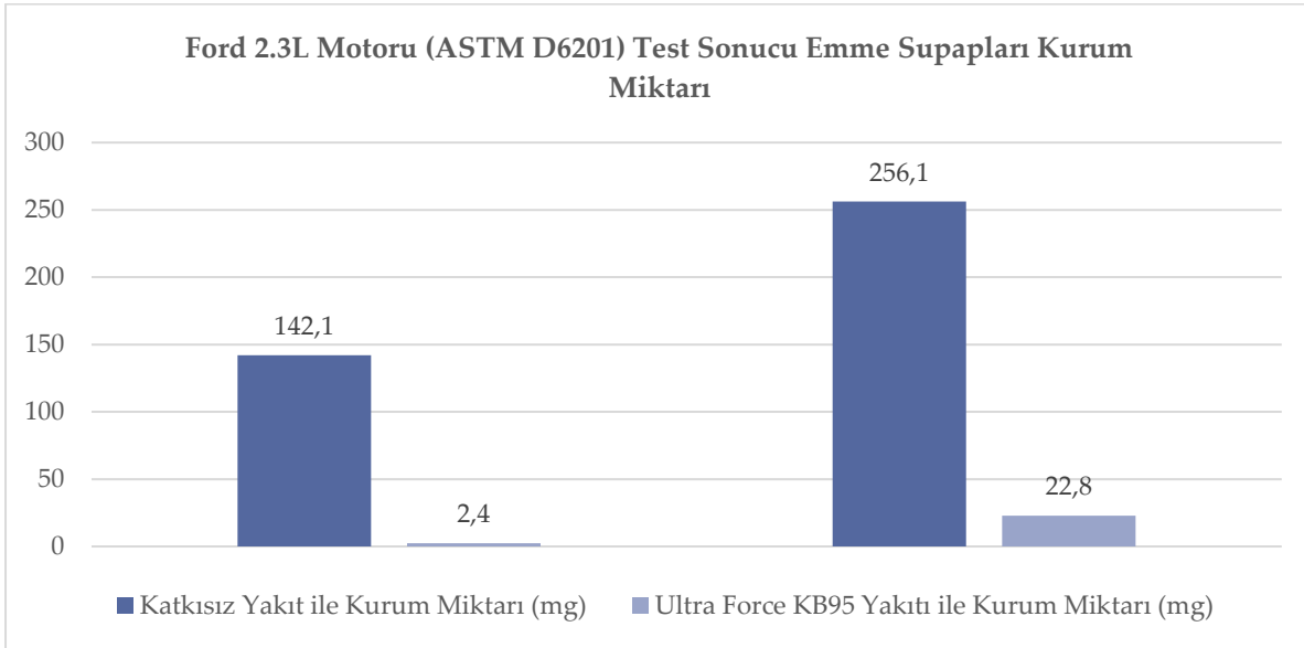
Ŗekil 1 Katkısız KB 95 ve OPET Ultra Force 95 katkılı yakıtlar kullanılarak Ford 2,3-L motoru ile 100 saatte yapılan temiz tutma testi.
