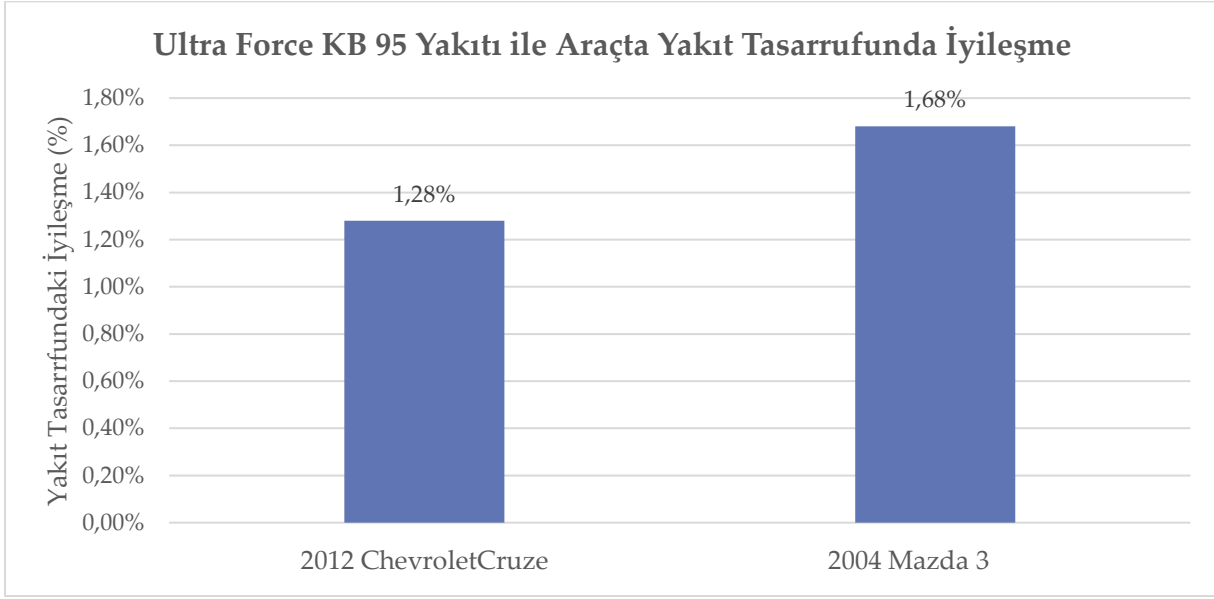
Şekil 6 Yakıt Tasarrufundaki İyileşme (Otoyol test sürüşü).
