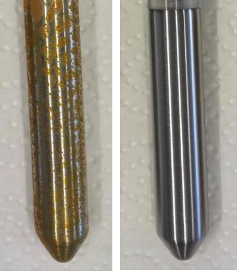
Şekil 5 Katkısız KB 95 (sol) ile ULTRA FORCE 95 Katkısı ile hazırlanmış benzin (sağ) karşılaştırmalı laboratuvar korozyon testi.
